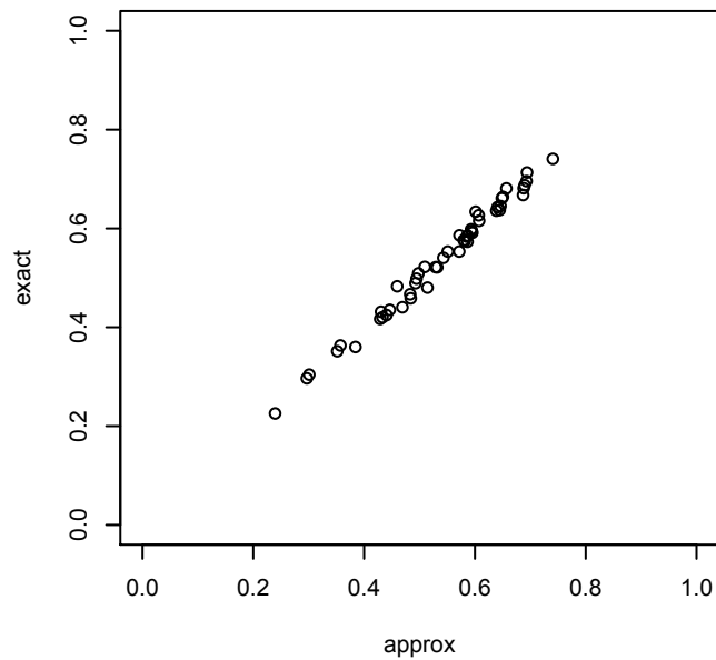
chunks=5, L=5
