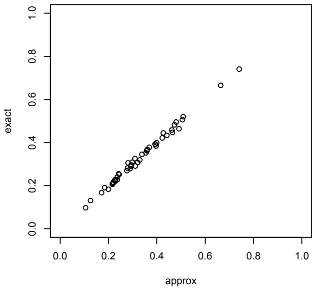
chunks=1, L=10
