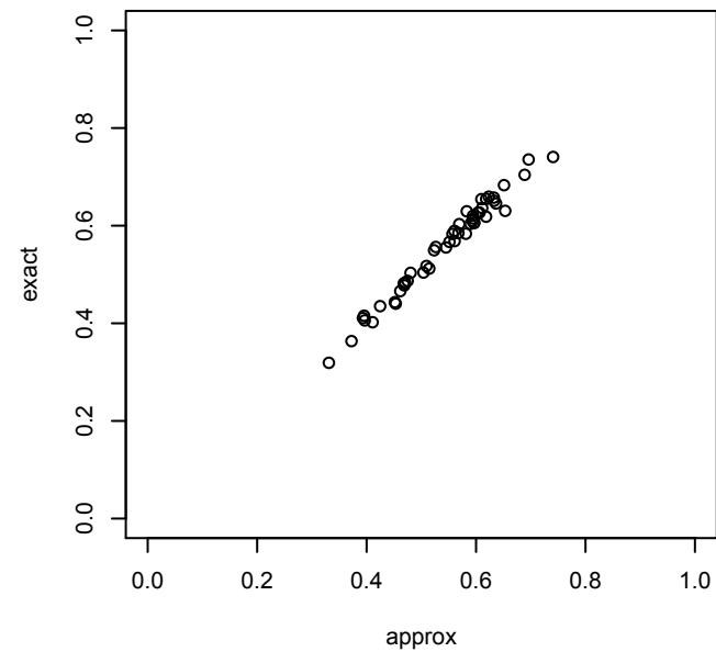
chunks=7, L=5
