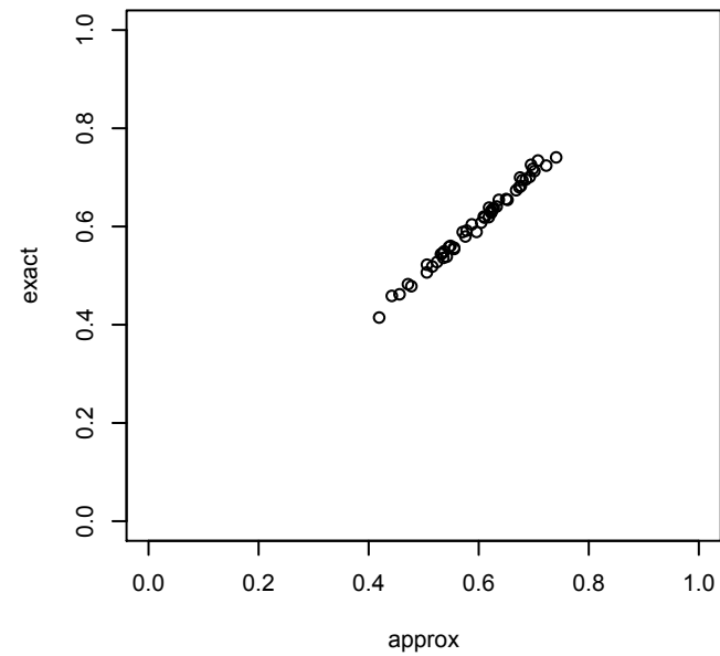
chunks=5, L=10
